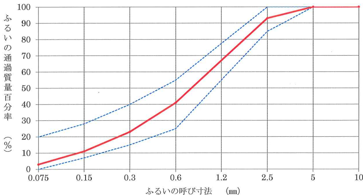
粒度曲線図
