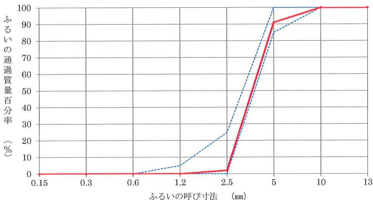
粒度曲線図
