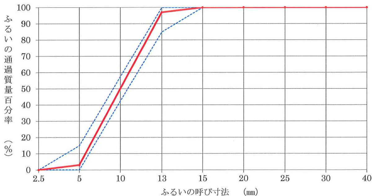
粒度曲線図
