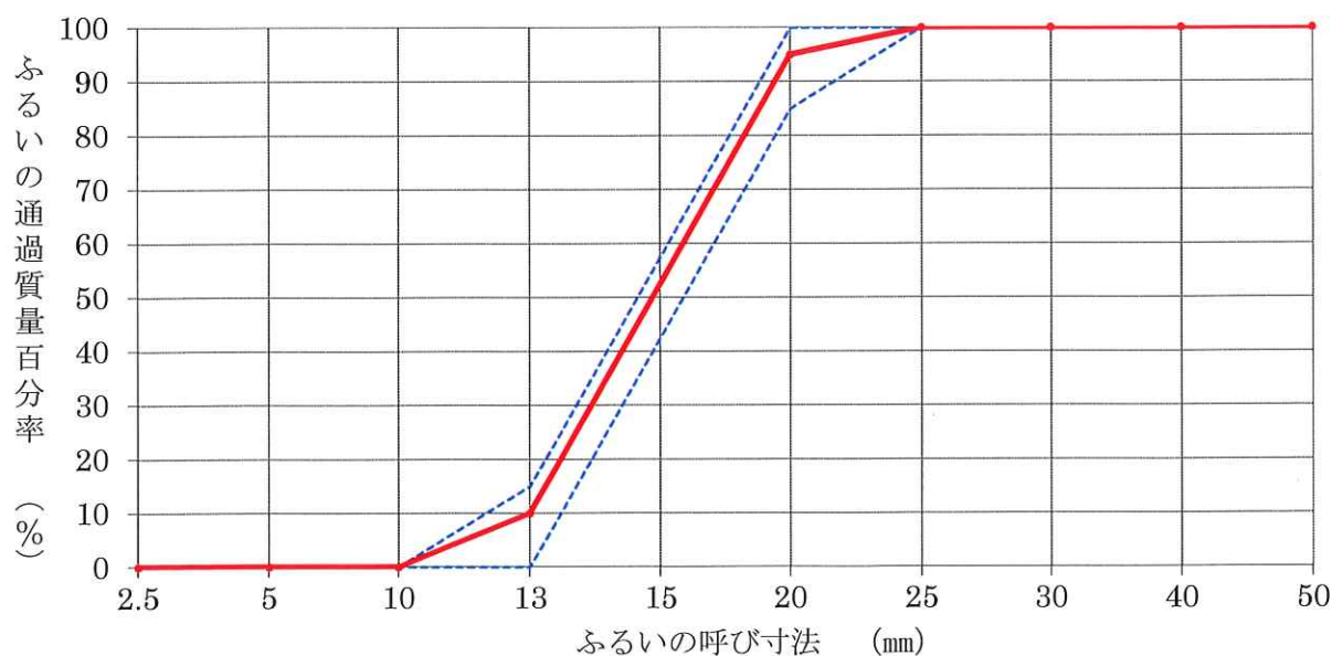
粒度曲線図
