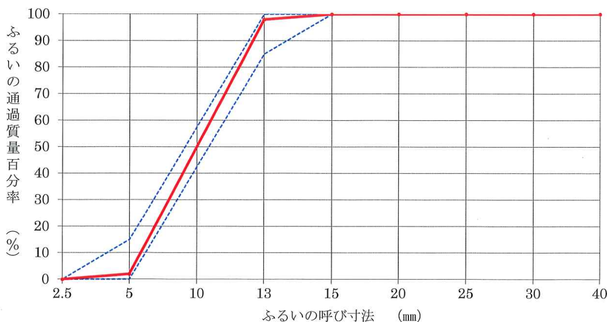
粒度曲線図
