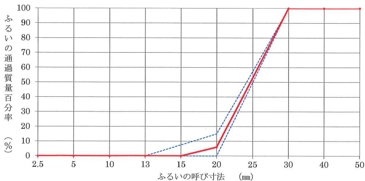
粒度曲線図
